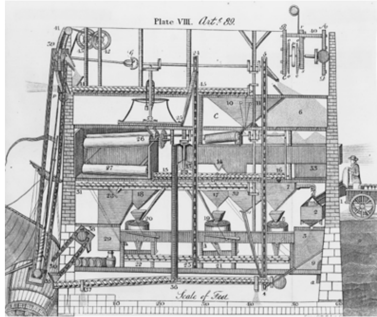
Dönemin buharlı un fabrikasının teknik çizimi.
